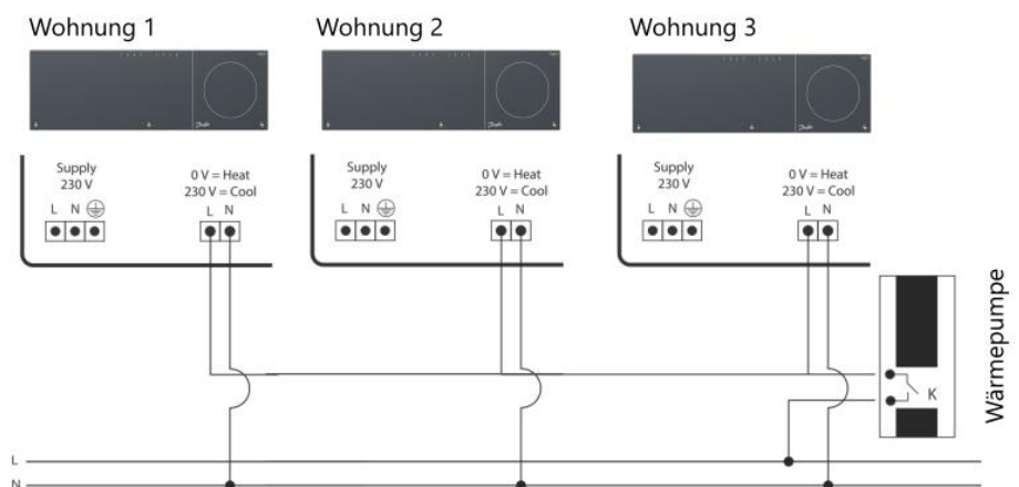
Anschluss von mehreren Regelverteiler im selben Gebäude
